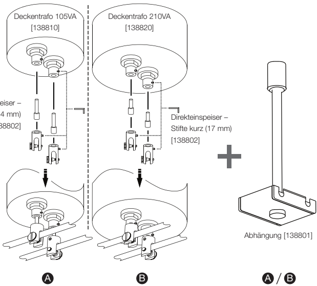
Anschlussbeispiel mit Direkteinspeiser [138802]
